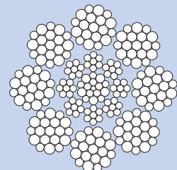
Fig. 22: DRAKO 250 T, 8x19W + IWRC
