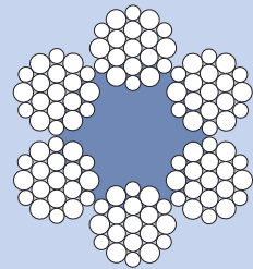
Fig. 19: 6x19W + NFC
