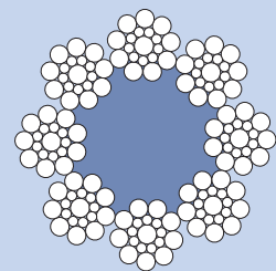
Fig. 20: 8x19S + NFC
