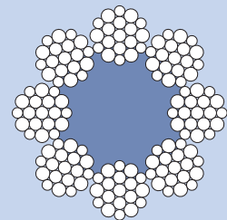
Fig. 21: 8x19W + NFC
